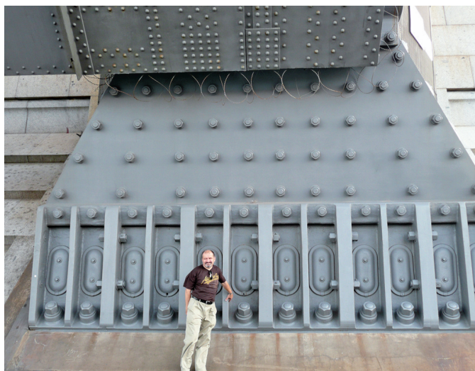
Autor artykułu na tle mostu, postać człowieka umożliwia ocenę wielkości przegubu łuku
